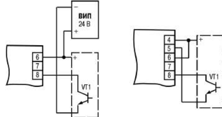
Рисунок 5.4 – Подключение активных датчиков с n-p-n -выходом: 1) при работе от ВИП; 2) при работе от внутреннего ИП
