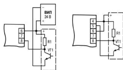
Рисунок 5.3 – Подключение пассивных датчиков с n-p-n -выходом: 1) при работе от ВИП; 2) при работе от внутреннего ИП
